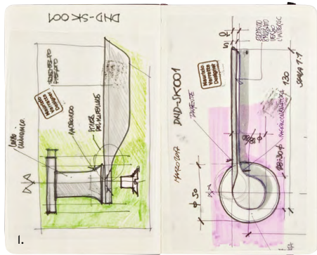
1. Эскиз ручки Levante в блокноте – Study for levnte lever on notebook
